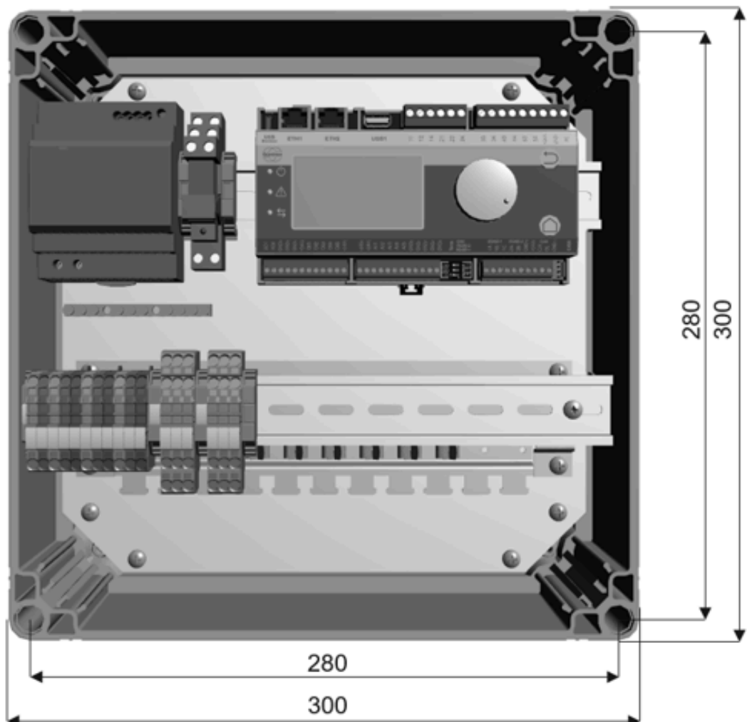
Maßbild Gehäuse aicore fusion
